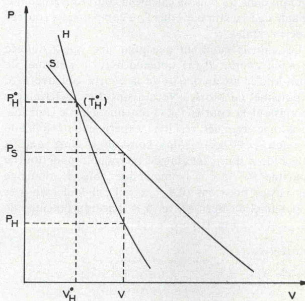
FIG. I. — Détermination de l'isentropique P_S passant par un point donné ( P_H^0, V_H^0, T_H^0 ) de la courbe de Hugoniot P_H .
